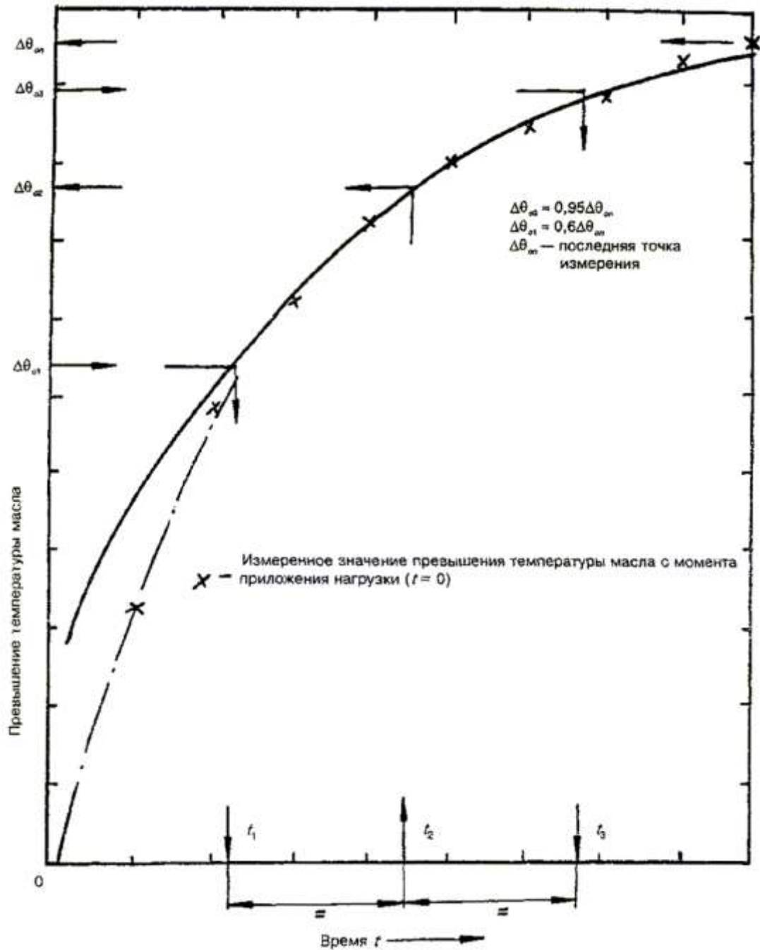
Рисунок В.2 - Определение действительной постоянной времени масла \tau_o по кривой превышения температур
