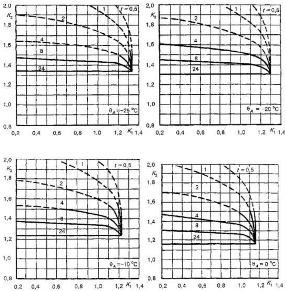
Рисунок 10 - Трансформаторы средней и большой мощности с охлаждением ОН . Допустимые режимы нагрузки с нормальным сокращением срока службы
